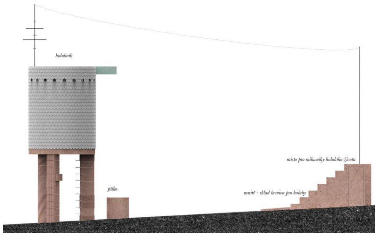
pohled jihovýchodní
